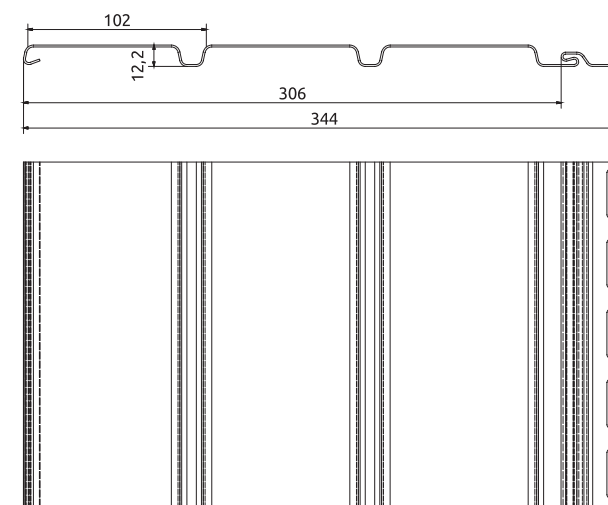
Panel podstawowy (pełny)
