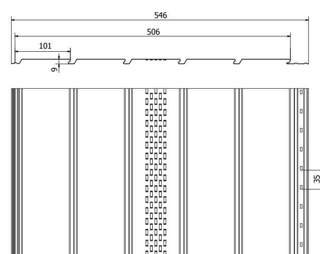
Panel wentylacyjny (perforowany)
