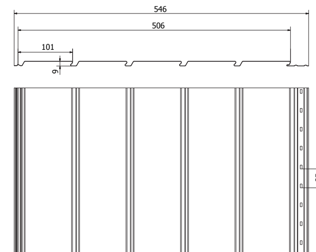
Panel podstawowy (pełny)
